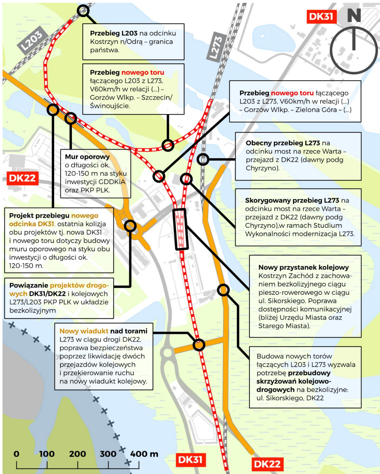
Rysunek 80 Konceptcja łącznicy oraz przebudowy układu drogowego w Kostrzynie nad Odrą
