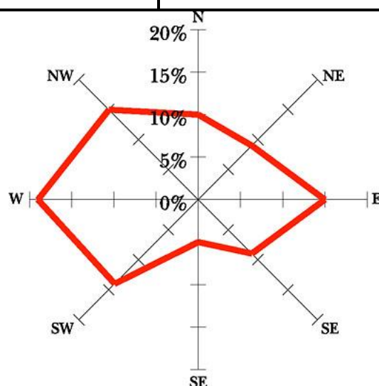
Ryc. 1 Wieloletnia „róża wiatru” dla Gorzowa.
